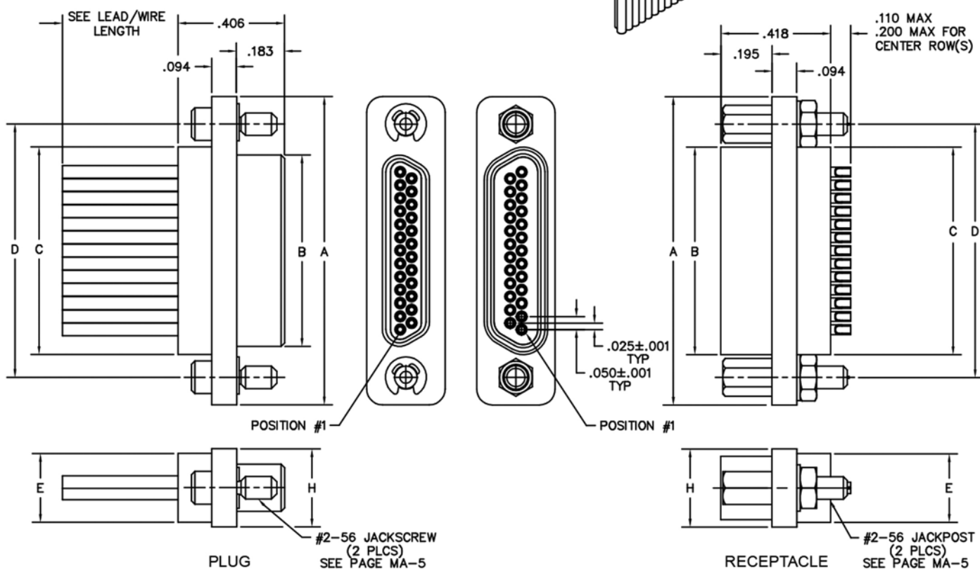
MMHT-212-025-161-41WA (METAL)
