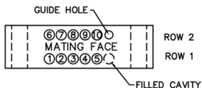
PLUG MA-211-010-161-A66WA
