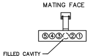
RECEPTACLE MA-141-005-261-A03WA
