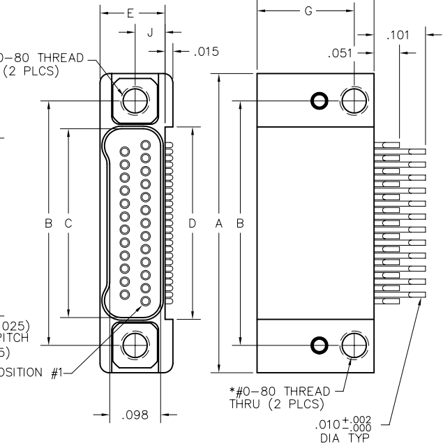
RECEPTACLE
