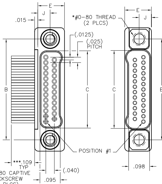
RECEPTACLE
