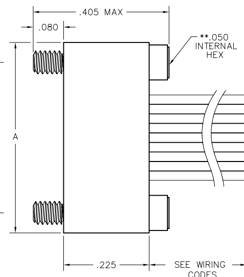
RECEPTACLE
