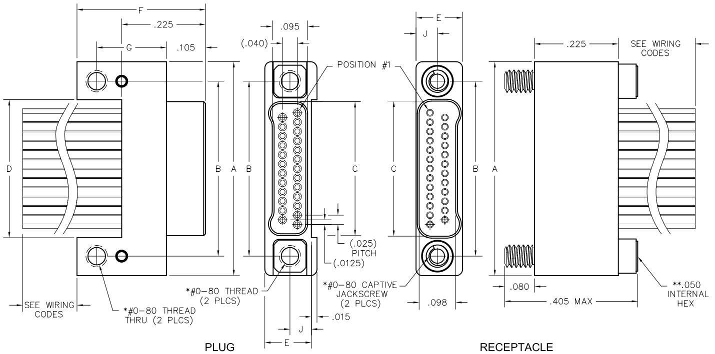
NM-222-025-261-JCAC (METAL)
