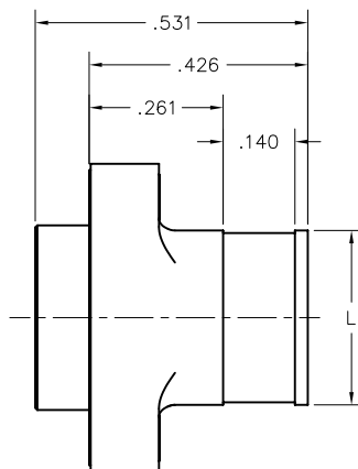
RECEPTACLE
