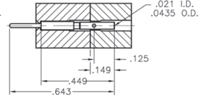
28-30 AWG
