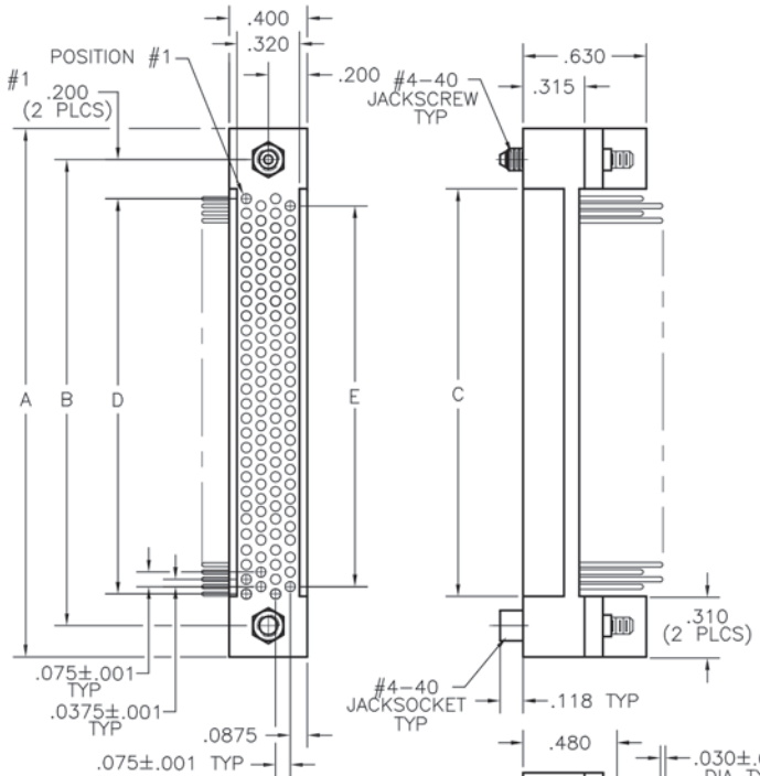
RECEPTACLE
